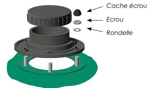
Trappe de visite
